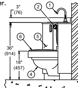
MODEL# 4044-R-1
