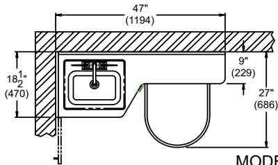
MODEL# 4044-R-3
