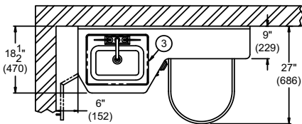
MODEL# 4044-R-3
