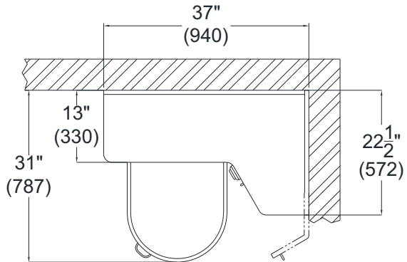
MODEL# 4040-L-2-FCI
