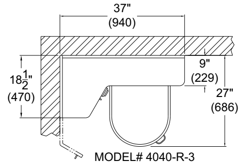
MODEL# 4040-R-3
