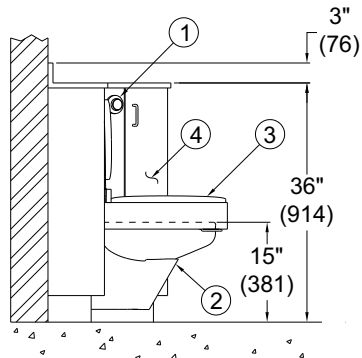
MODEL# 4040-L1
