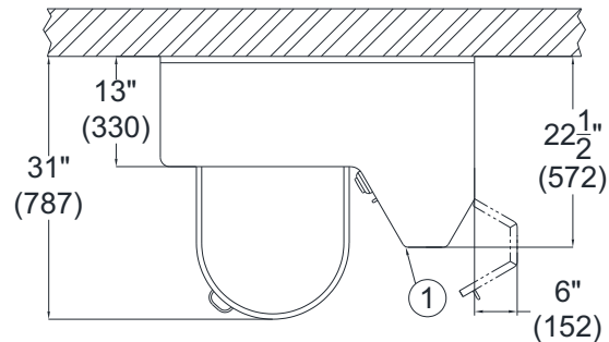
MODEL# 4040-L1-FCI
