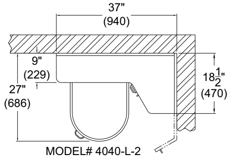
MODEL# 4040-L-2
